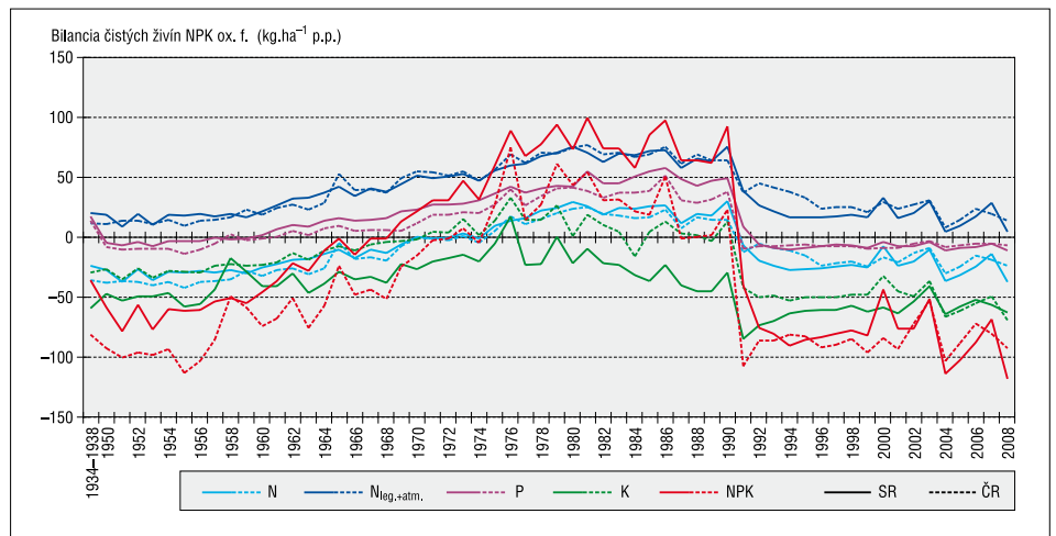
Obr. 4. Časová bilancia čistých živín NPK – SR a ČR
