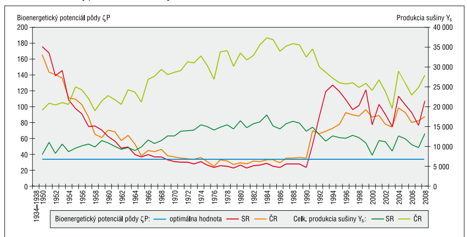
Obr. 5. Optimálna hodnota a časový vývoj bioenergetického potenciálu pôdy a časový vývoj celkovej produkcie sušiny – SR a ČR
